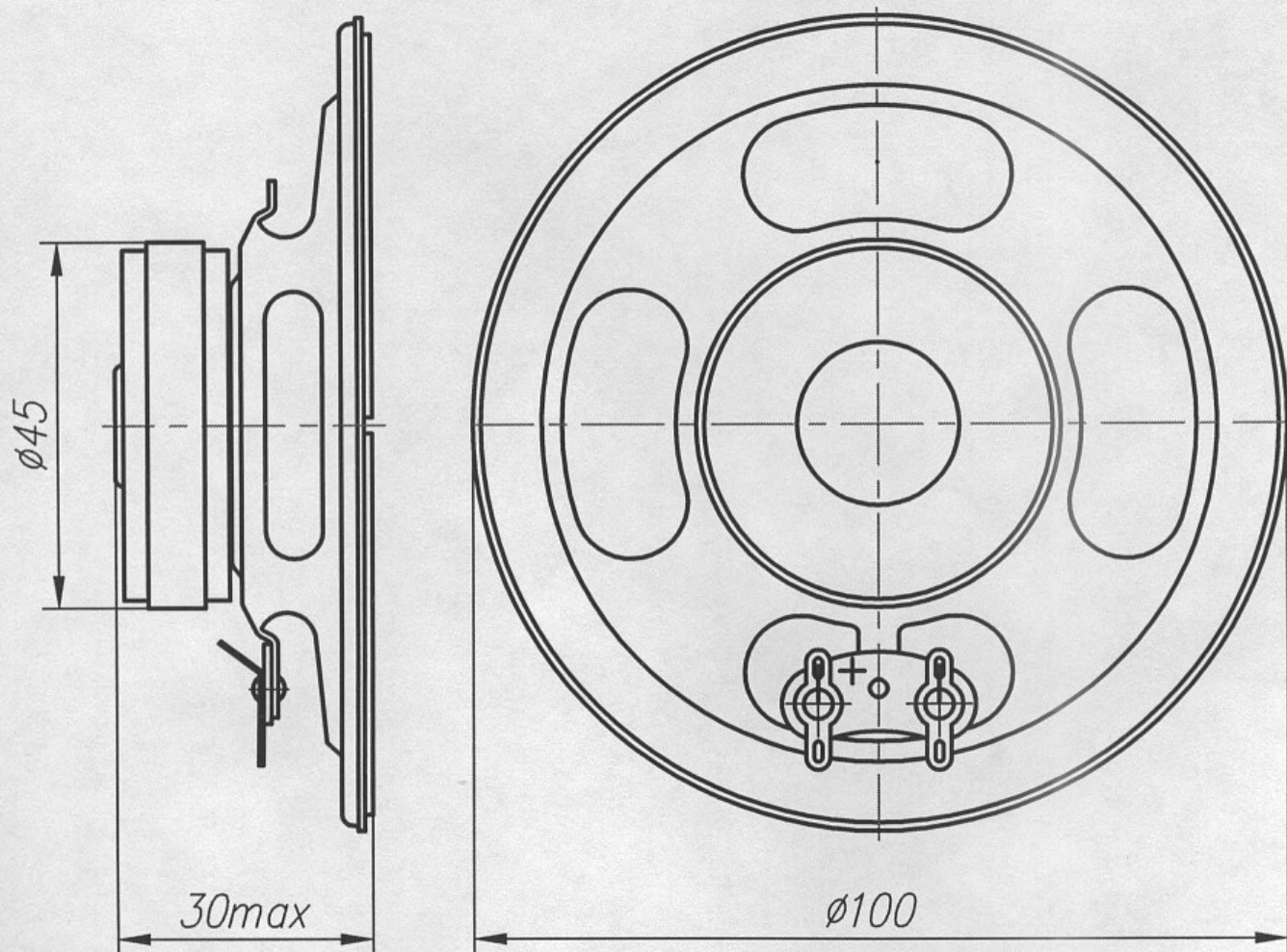
Головка громкоговорителя 3ГДШ-16
