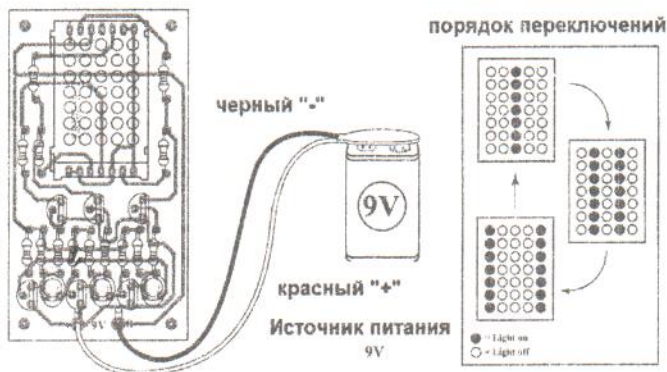
Рис.3 Схема подключений
