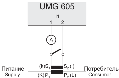
Рис. Пример, измерение тока через дополнительный амперметр.
