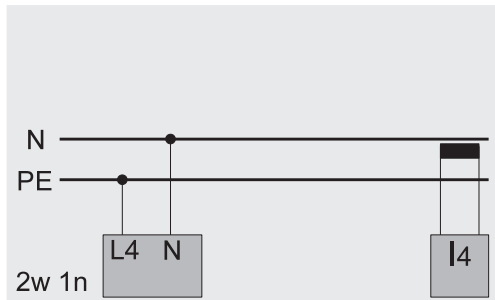
Рис. Измерение напряжения между N и PE. Измерение тока на нейтрали.
