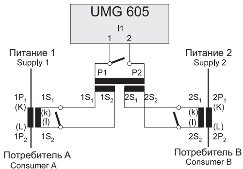
Рис. Пример подключения, измерение тока через трансформатор суммарного тока.
