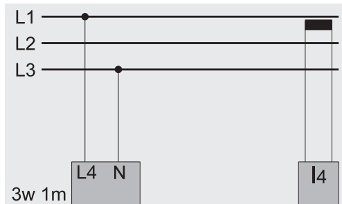
Рис. Измерение в трехфазной 3-проводной сети с симметричной нагрузкой.
