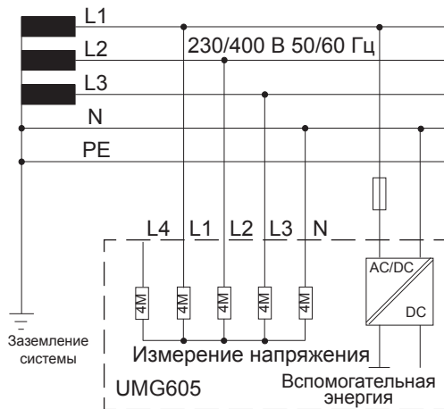
Рис. Принципиальная схема, UMG605 в TN-сети.
