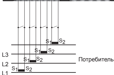
Рис. Пример подключения, измерение тока через трансформатор тока.
