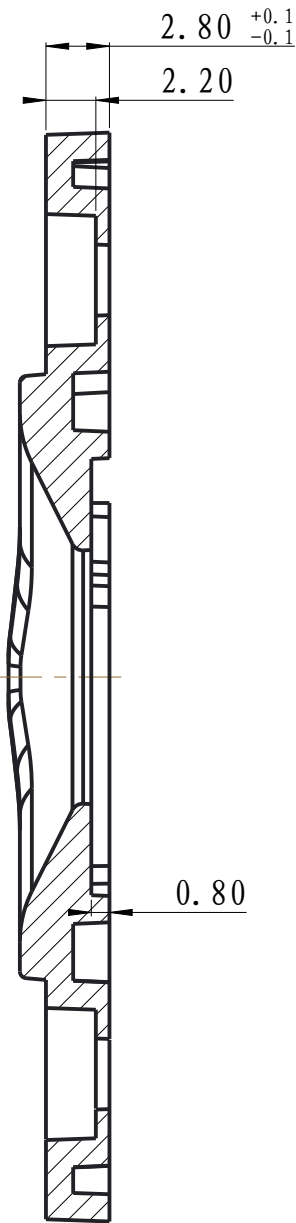
截面 XSEC0001-XSEC0001
