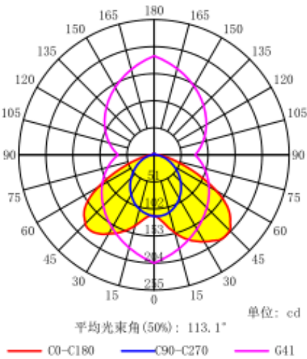
配光曲线
