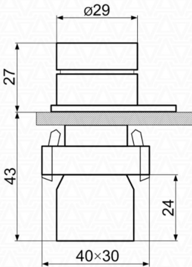
Размеры поворотного переключателя серии 3SA8-BD
