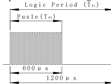
图 4 低电平脉宽、逻辑周期宽度
