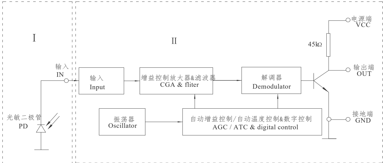
图 5 内部框图 Figure5 Block diagram
