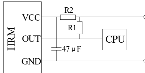
图 12 推荐电路 Figure12 Recommended Circuit
